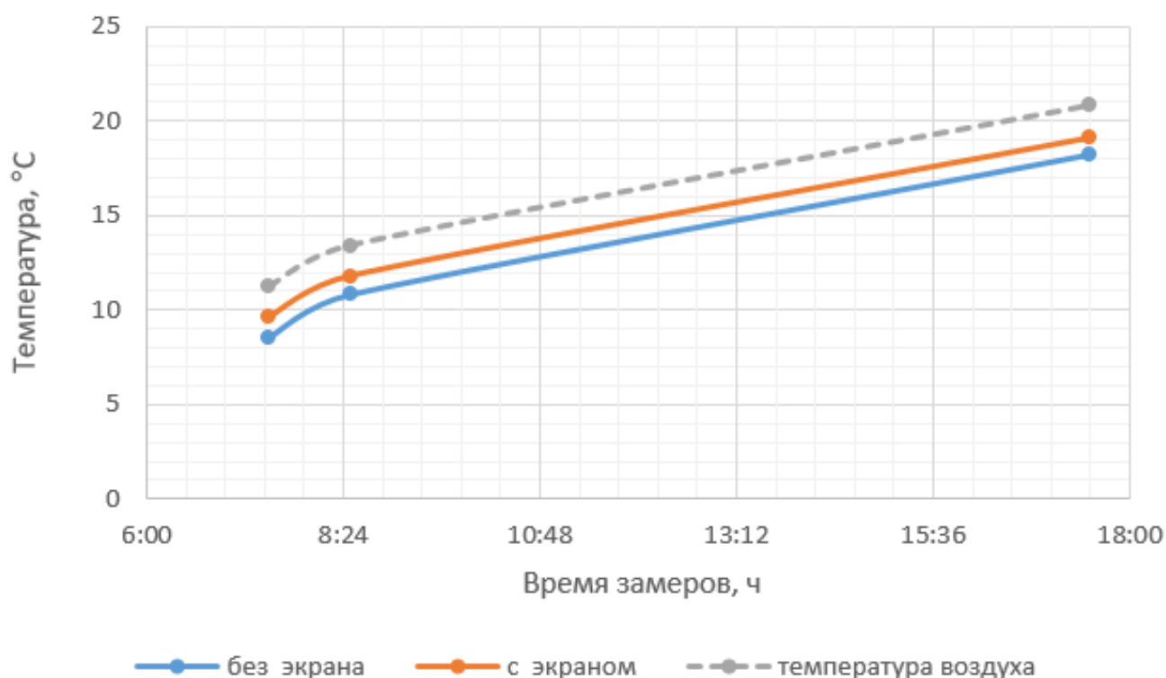
Рис. 3. Изменение температуры поверхности стены (сайдинг) с «зелёным» и без «зелёного» экрана в сентябре
