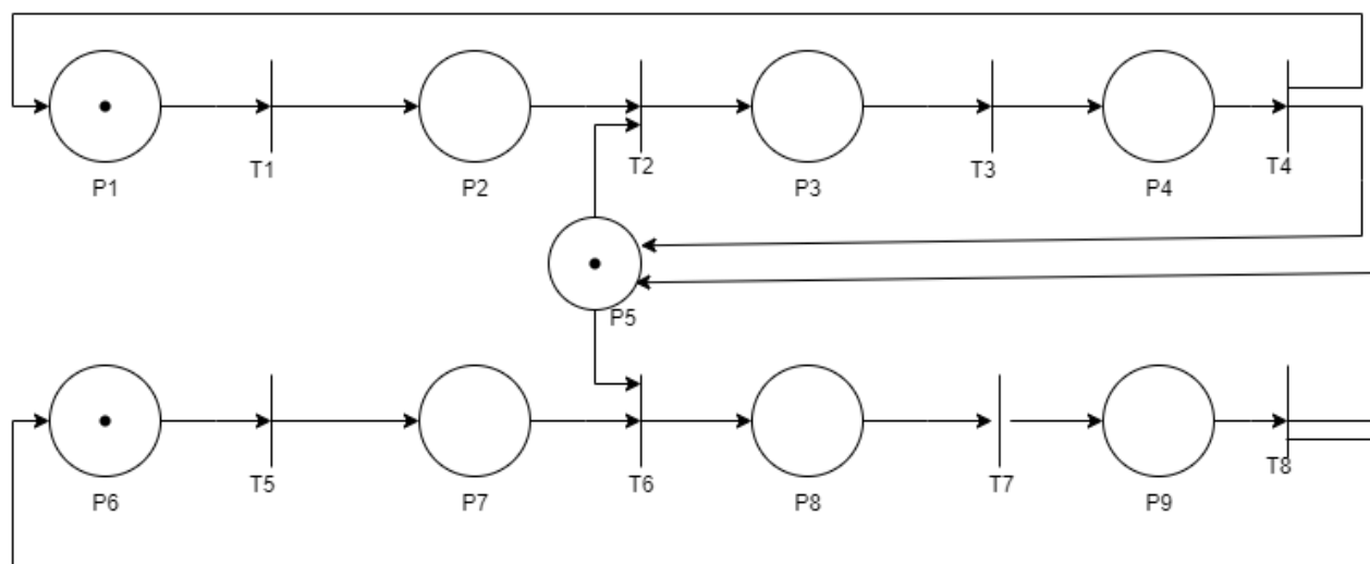
Рис. 1. Сеть Петри
