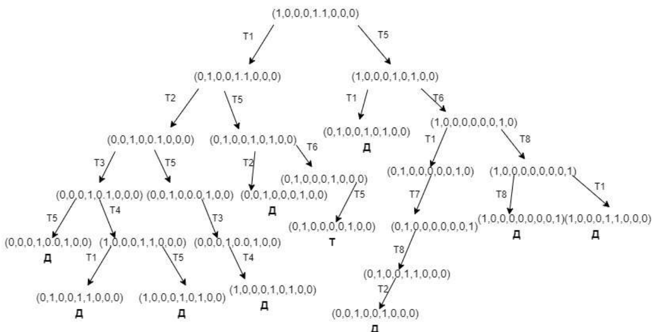
Рис. 2 . Дерево достижимости
