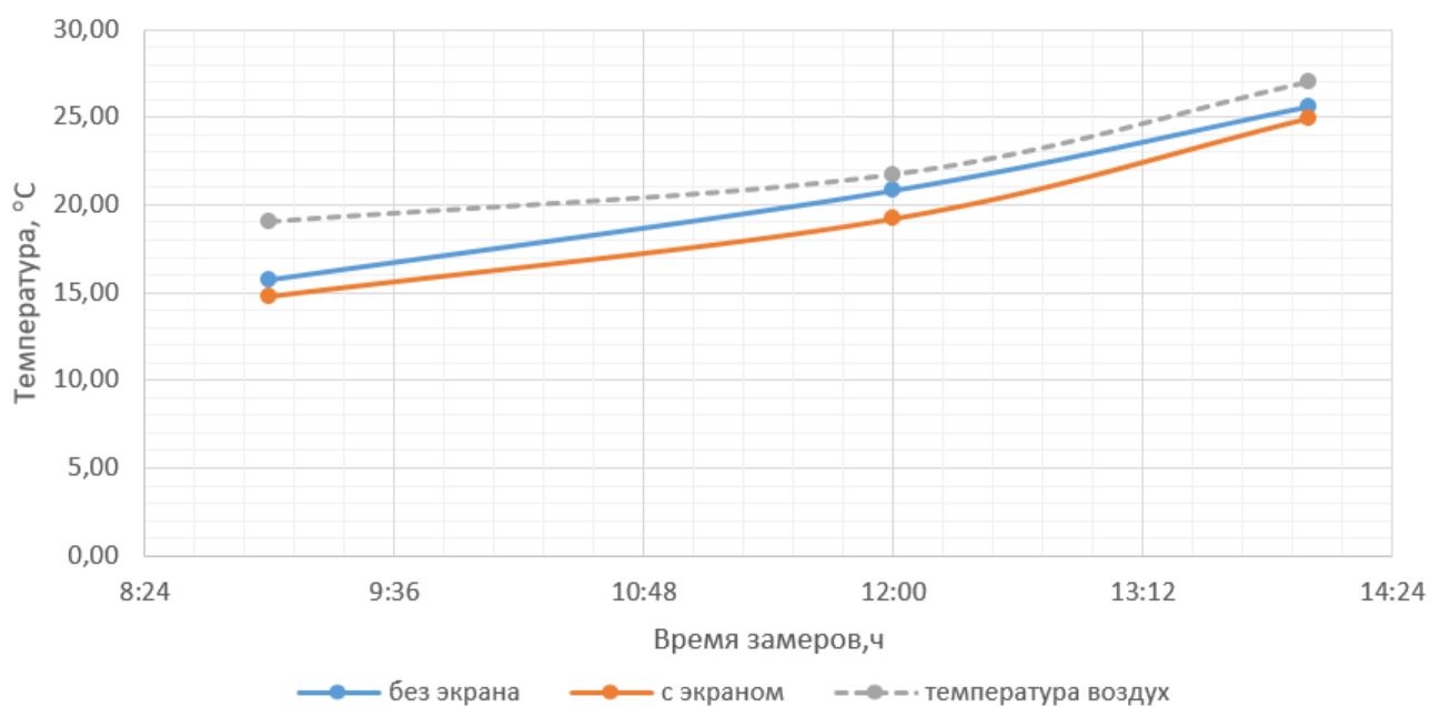
Рис. 2. Изменение температуры поверхности стены (сайдинг) с «зелёным» и без «зелёного» экрана в мае
