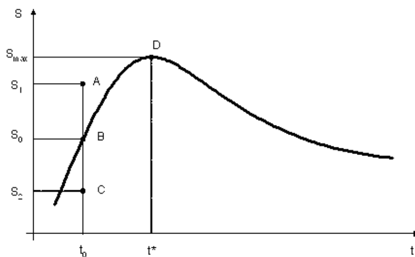
Рисунок 1. Модель кредитного портрета потенциального заемщика.
