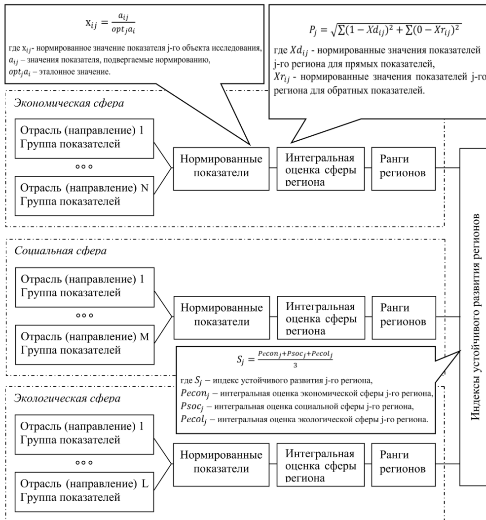
Рисунок 2 – Алгоритм расчета индексов устойчивого развития субъекта
