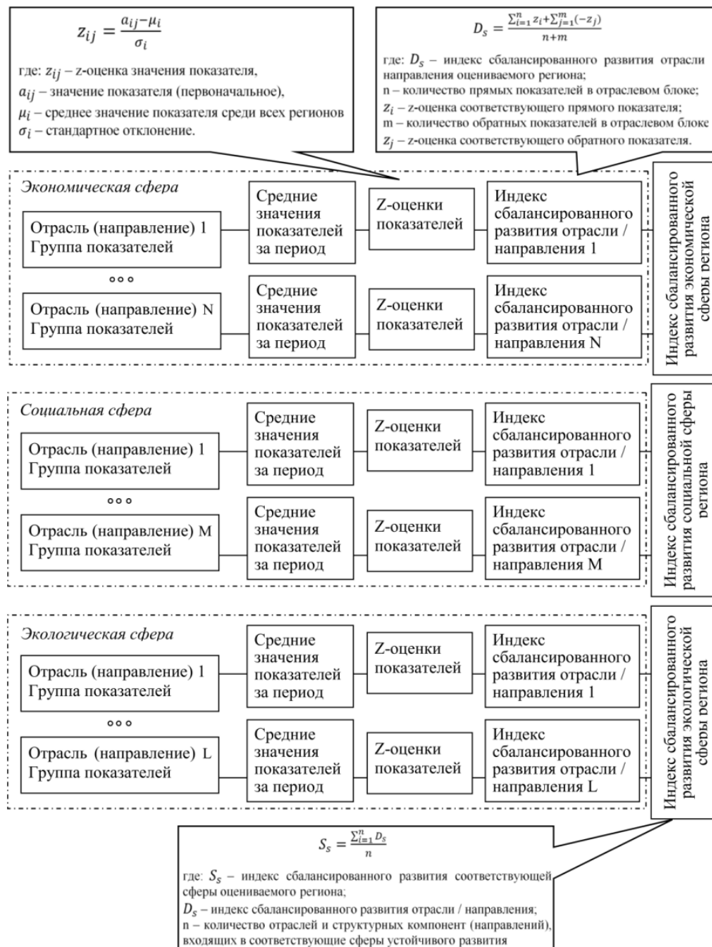
Рисунок 3 – Алгоритм расчета индексов сбалансированного развития сфер региона
