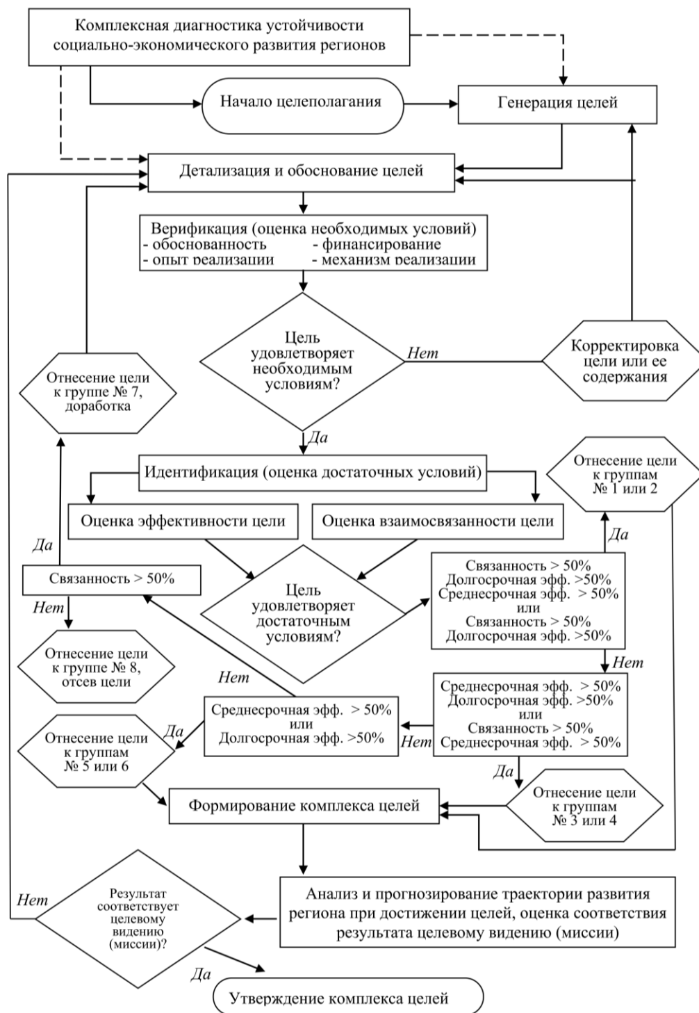
Рисунок 6 – Алгоритм отбора и приоритизации целей региональной экономической политики устойчивого развития
