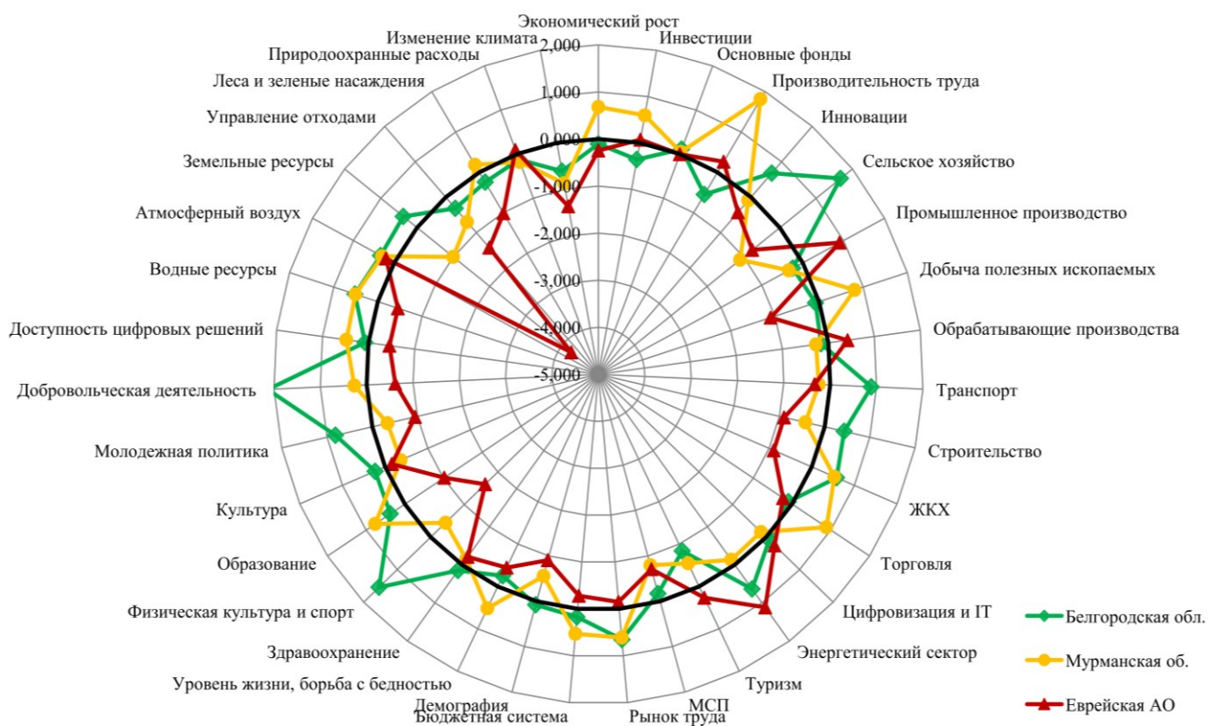
Рисунок 5 – Детализированное сравнение сбалансированности развития модельных регионов
