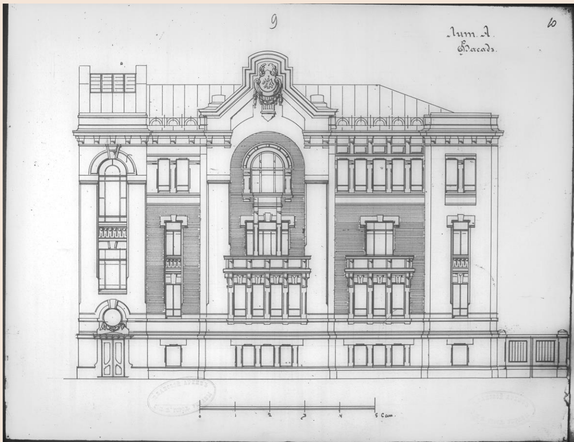
Проект фасада флигеля Менделеева в 4 этажа, Б. Пушкарская ул. ,д. 28, арх. А. И. фон Гоген. Лит. А. © ЦГИА СПб. Ф. 513. Оп. 1. Д. 8369. Образ 11
