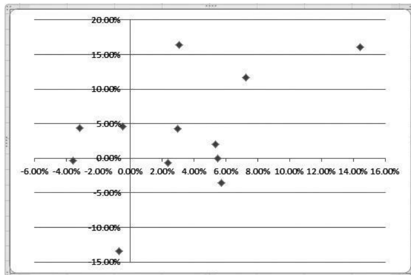
Рис. 1.39. Диаграмма рассеяния
