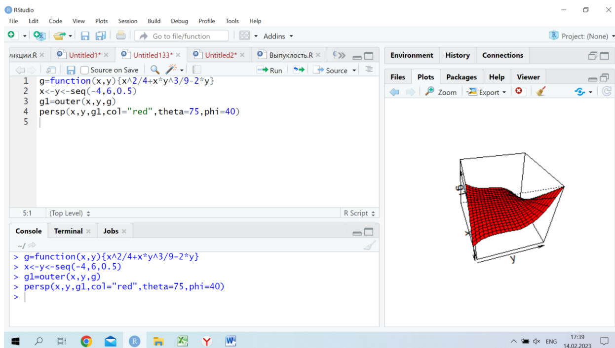
Рис.1 Код построения графика функции g = \frac{x^2}{4} + x \frac{y^3}{9} - 2y
