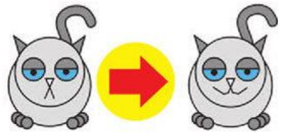
Динамические модели
