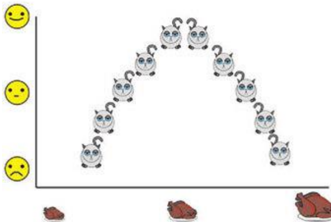
Нелинейная модель
