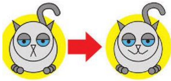
Статические модели
