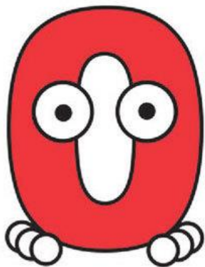
Нулевая гипотеза
