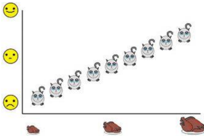
Линейная модель
