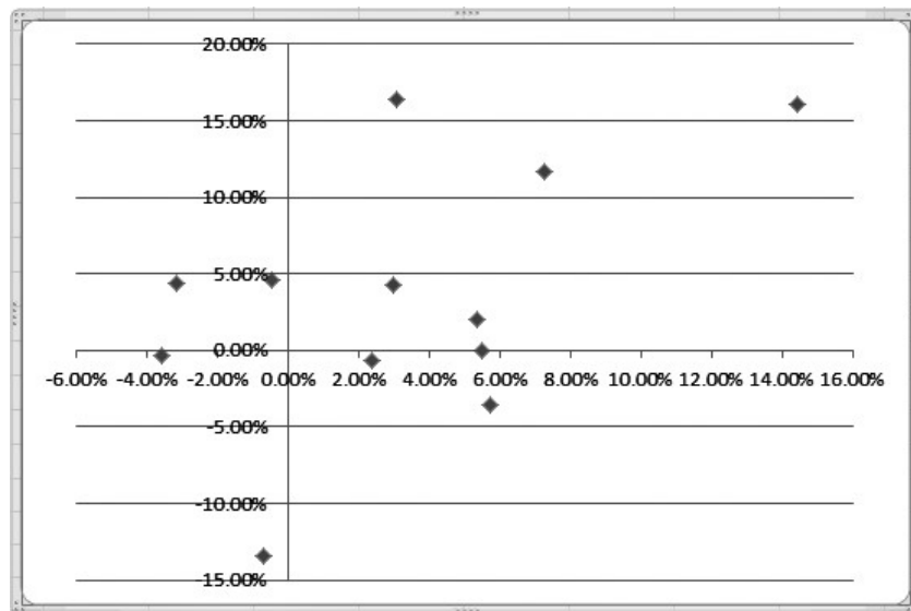
Рис. 1.39. Диаграмма рассеяния
