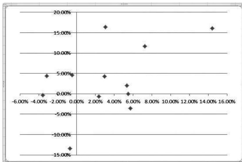
Рис. 1.39. Диаграмма рассеяния
