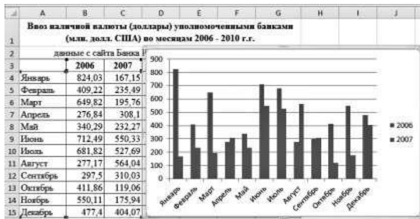
Рис. 1.33. Созданная гистограмма
