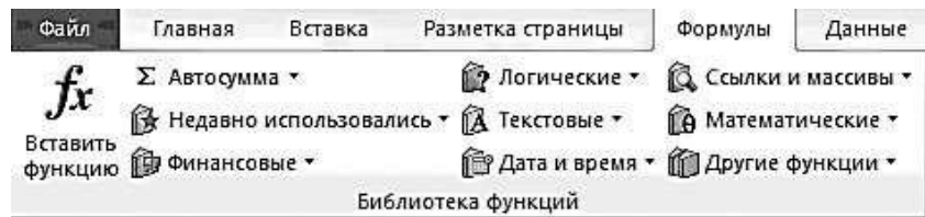
Рис. 1.1. Библиотека функций
